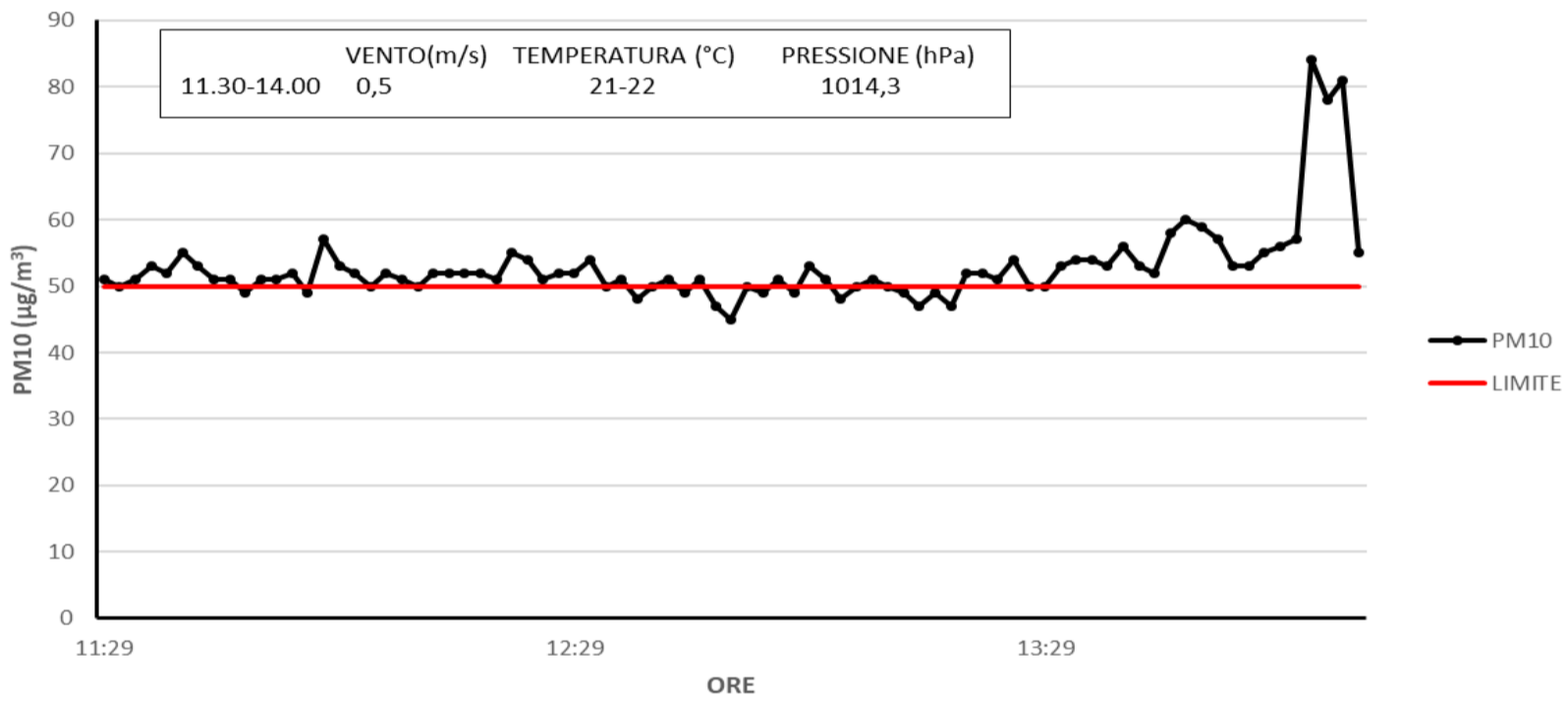
RILEVAMENTO PARTICOLATO 16/04/18- ZONA PARCHEGGIO MOTORINI (ORE 11:27-14:09)
